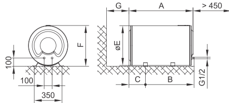
SI. 2: Ležeča namestitve na tla
