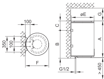
SI. 1: Pokončna namestitve na steno
